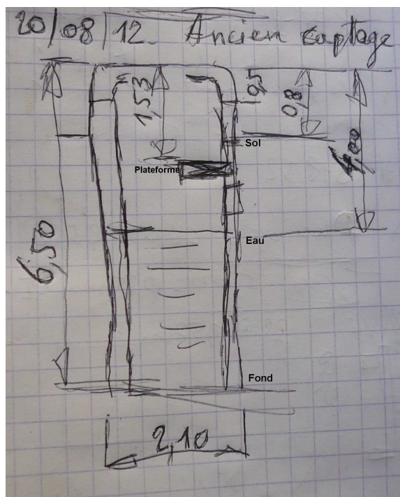
(plan à main levée du captage de 1914 avec ses dimensions- 2012)
