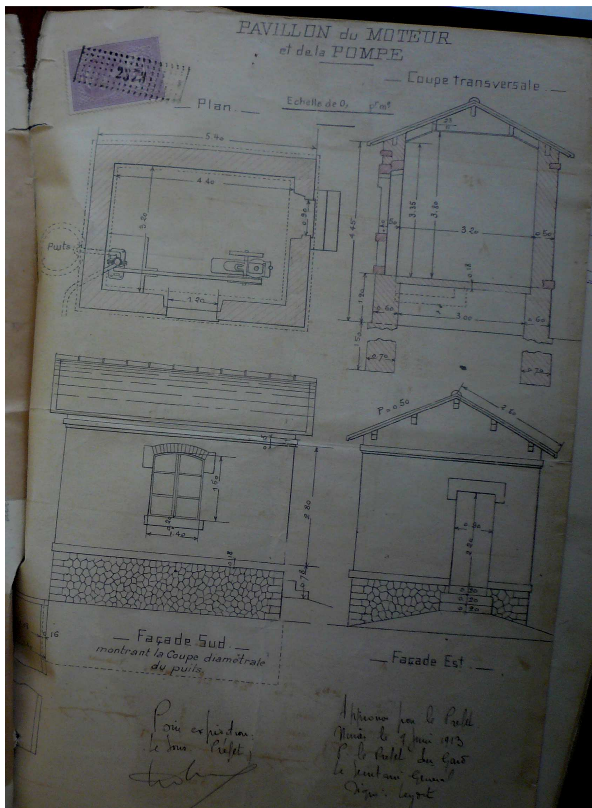
Pavillon sur l'Alzon-Les Moutes - Plan d'origine et réinterprétation pour une meilleure visibilité en version papier
